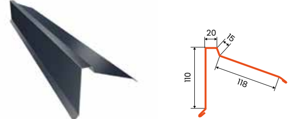
PHR terminație de acoperiș cu o singură înclinare
