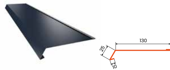
bordură de streășină dreaptă PHR
