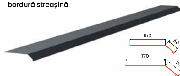
bordură streășină
