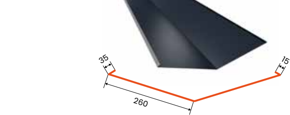
streășină de coș PHR
