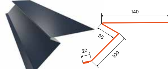
bordură streășină trapezoidală mare PHR
