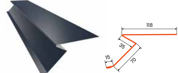
bordură streășină trapezoidală PHR
